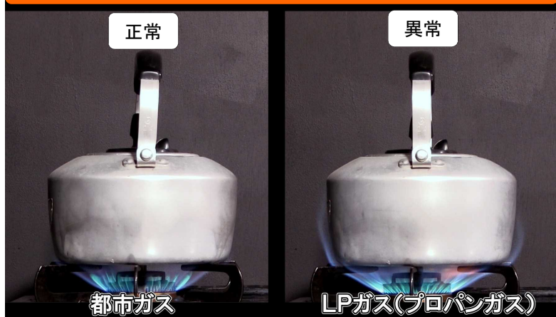
都市ガスとLPガスを供給して燃焼状態を比較
