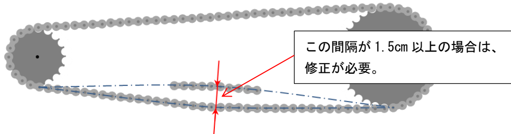
図8 チェーンのたるみの判別法（外装変速機なしの場合）
