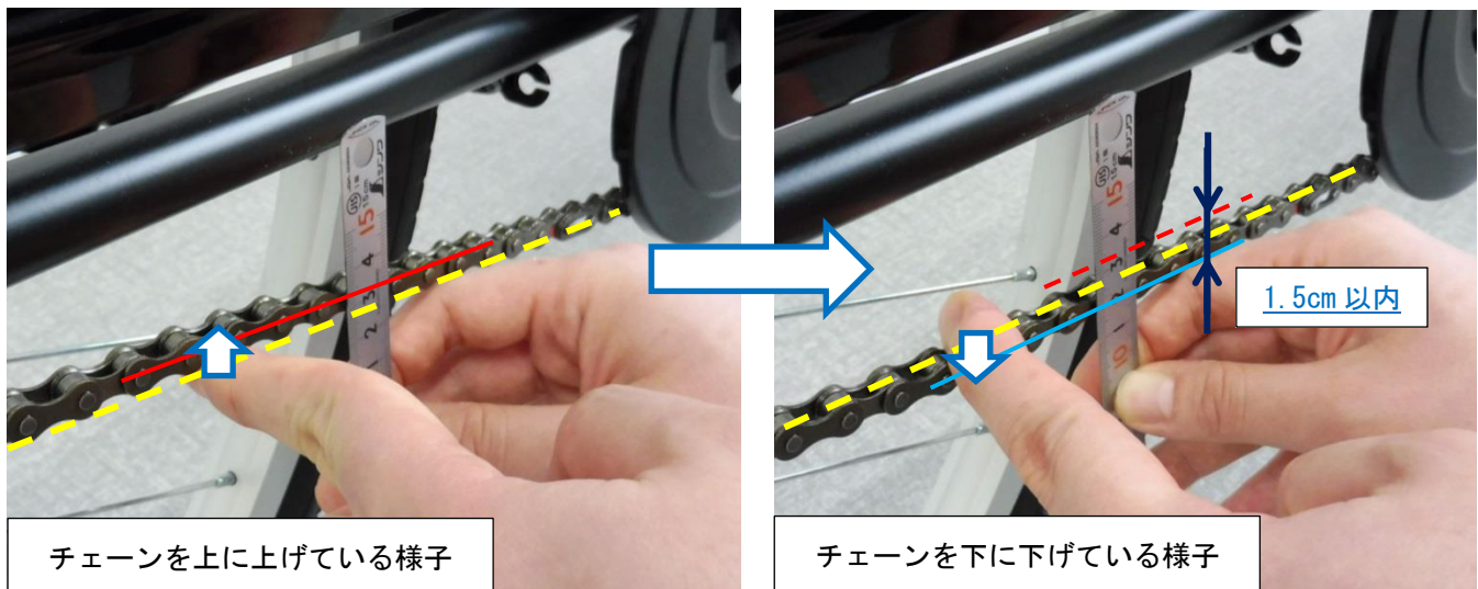
(写真6) チェーンのたるみを判別している様子
