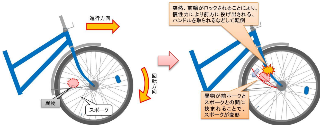
図 7 異物を巻き込んでスポークが変形する状況
