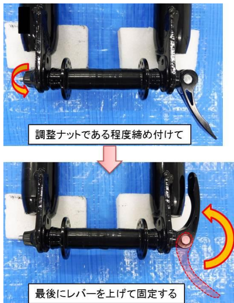
(写真 3) クイックリリース方式の正しい固定方法
