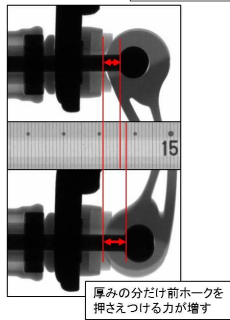
(写真 4) レバー開放時（上）とレバー固定時（下）
