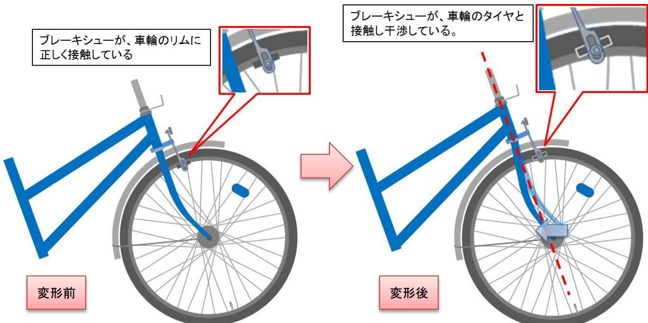
図 9 前ホークが変形してブレーキシューがタイヤと干渉する状況
