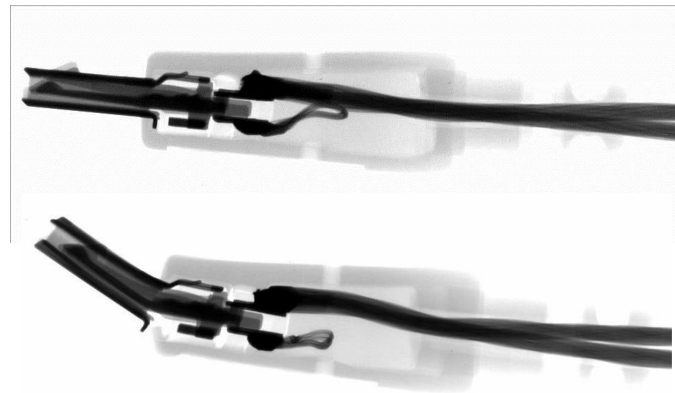
正常なマイクロUSB(上)と力を加えて折れ曲がったマイクロUSB(下)。内部のコネクタピンが変形しています
