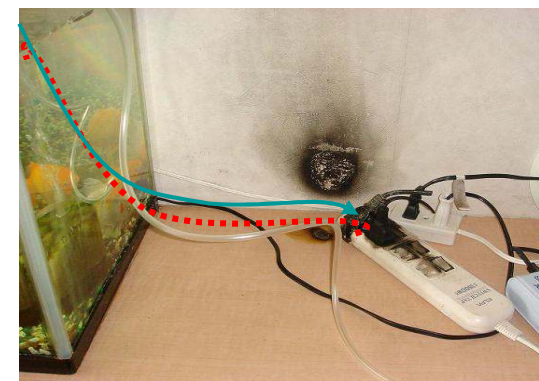
..... 電話機電源コード配線経路 → 水槽水の流れ経路
