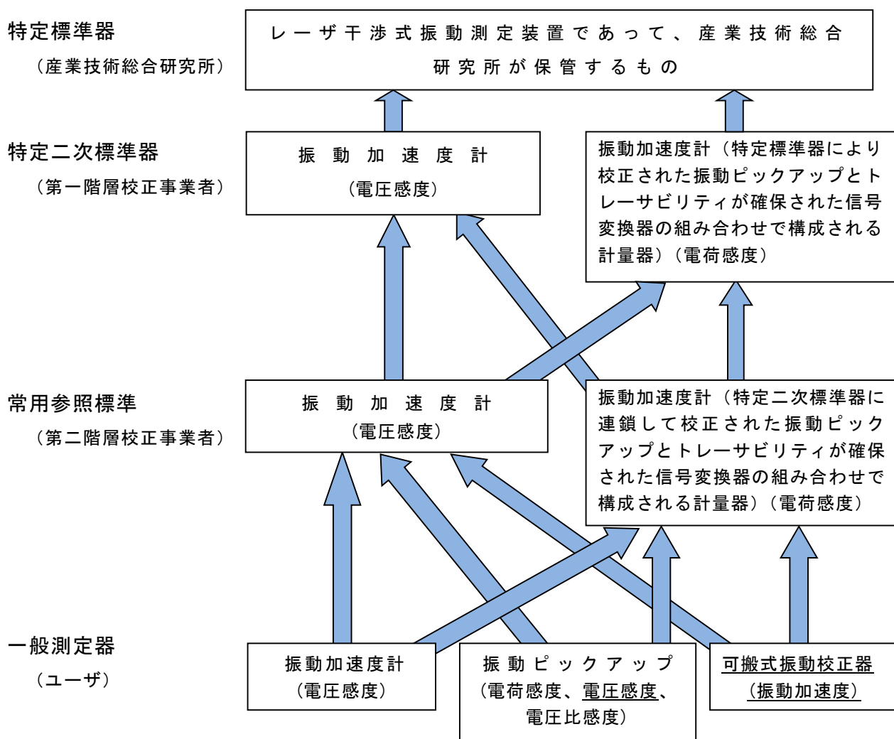
図1 トレーサビリティ体系図(例示)
