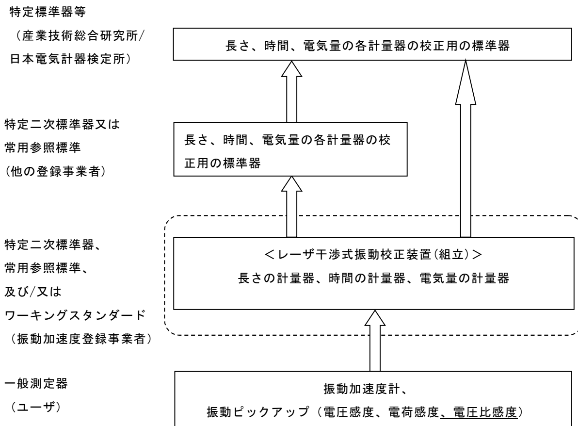
図2 レーザ干渉式振動校正装置(組立)トレーサビリティ体系図(例示)
