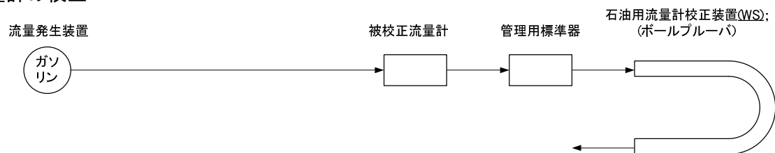
図 4 試験液種の拡張方法: 特定二次標準器と液種拡張用機器(石油用流量計)を用いる場合
